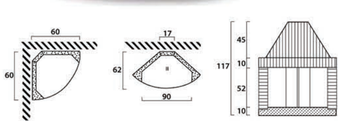
C PRISMATO angolare
